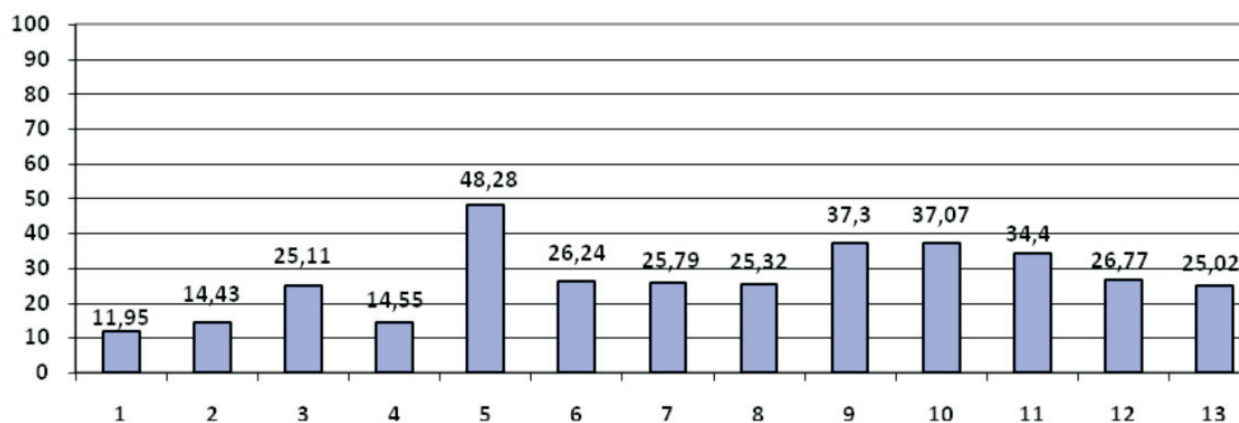
Рис. 1. Доля видового состава растений флористических округов Дагестана (1 – Примор., 2 – Тер.-Кум., 3 – Тер.-Сул., 4 – Сам., 5 – Предг., 6 – Казб., 7 – Буйн., 8 – Кайт.-Таб., 9 – Центр.-Даг., 10 – Ахт.-Кюр., 11 – Дикл.-Дюльт., 12. – Бежг.-Дид., 13 – Транссам.)
